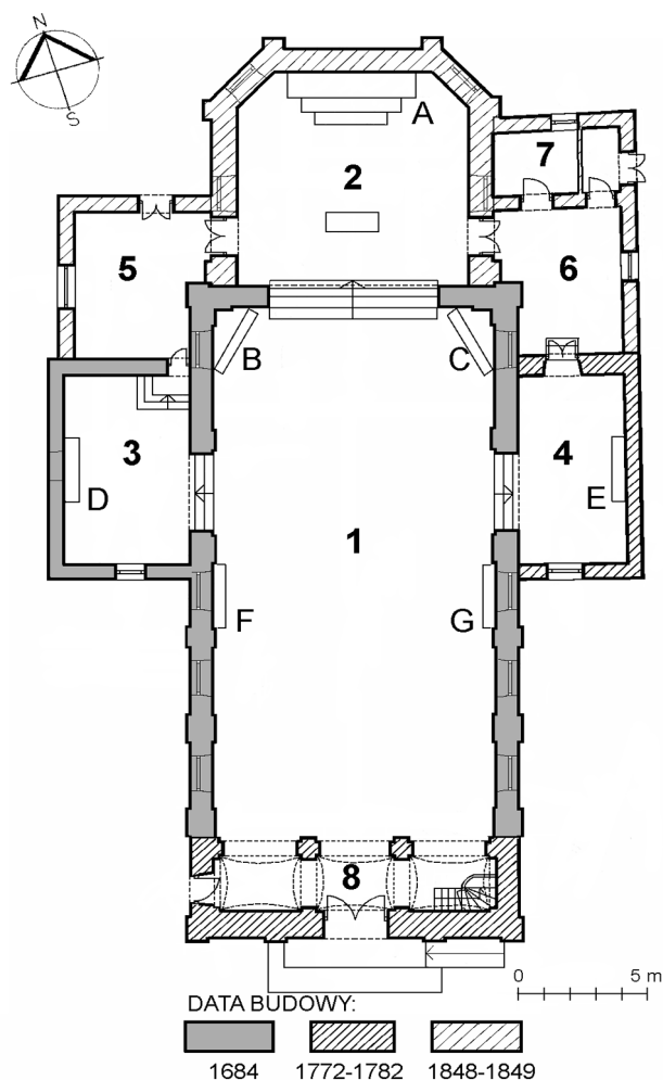
Rys. 1. Rzut przyziemia kościoła św. Piotra i Pawła w Żychlinie – etapy rozbudowy
