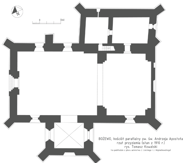
Rys. 1. Bożewo, kościół parafialny św. Andrzeja, rzut przyziemia, stan z 1910 r. (rys. Tomasz Kowalski, na podkładzie planu J. Lisickiego i J. Wojciechowskiego)
