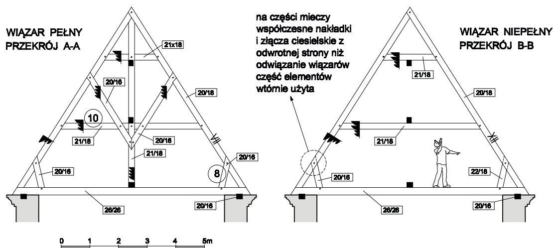
Wyniki badań architektonicznych więźby dachowej nad nawą i prezbiterium kościoła – przekroje poprzeczne. Rys. M. Warchoł
