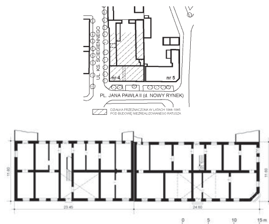
Rys. 5. Plan sytuacyjny i rzuty przyziemia budynków północnej pierzei d. Nowego Rynku ob. Pl. Jana Pawła II nr 3 (d. nr 4) i 4 (d. nr 5). Oprac. autora wg rys. mgr J. Graczyk w karcie ewidencyjnej zabytków architektury i budownictwa z 1984 r., Ośrodka Dokumentacji Zabytków w Warszawie
