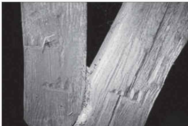
Ciesielskie znaki montażowe na elementach więźby. Fot. M. Warchoń
