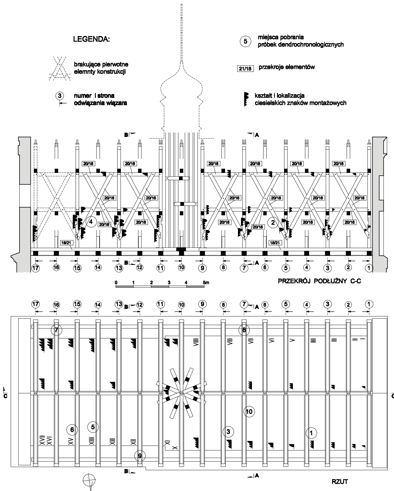
Wyniki badań architektonicznych więzby dachowej nad nawą i prezbiterium kościoła – przekrój podłużny i rzut dachu. Rys. M. Warchoń
