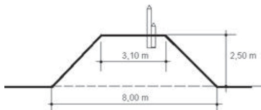
Rys. 3. Hipotetyczny przekrój wałów obronnych z częstokółem miasta lokacyjnego Zychlina. Oprac. autora. Objętość ziemi wałów o ogólnej długości około 800 m wynosi: [(8,0 + 3,1) : 2] \times 2,5 \times 800 = 11100 \text{ m}^3
