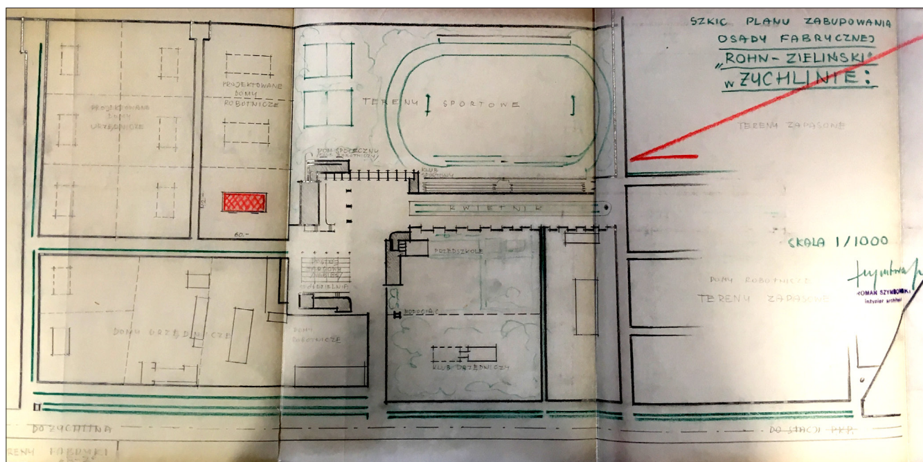
Rys. 3. Szkic planu zabudowania Osady fabrycznej „Rohn-Zieliński” w Żychlinie opracowany przez arch. R. Szymborskiego w sierpniu 1938 r. Budynek istniejący obrysowano cienką linią ciągłą, projektowane cienką linią przerywaną oraz grubą linią ciągłą z zaciemnieniem. Kratką oznaczono projektowany dla robotników budynek TOR. Archiwum Akt Nowych, zbiór BGK, Bank Gospodarstwa Krajowego w Warszawie, sygn. 2/235/0/11.3/2578
