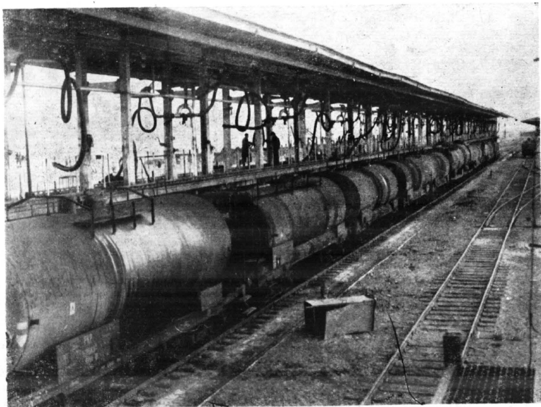
Kombinat — stacja nawleków. Napelnianie cystern produktem finalnym
