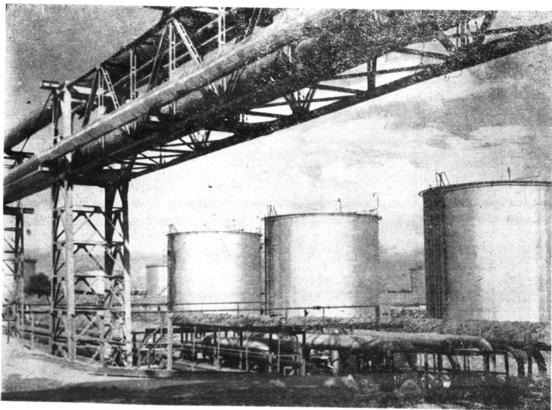
Kombinat — widok na zbiorniki manipulacyjne Reformingu
