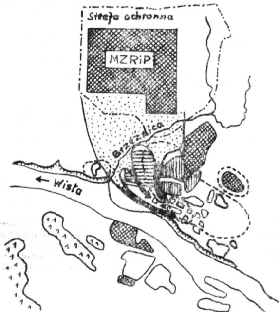
Rys. 7. Przestrzenny rozkład zanieczyszczeń w obszarze miasta Płocka (wg T. Kowalczyka, Notatki Płockie 1981, nr 2/107).
