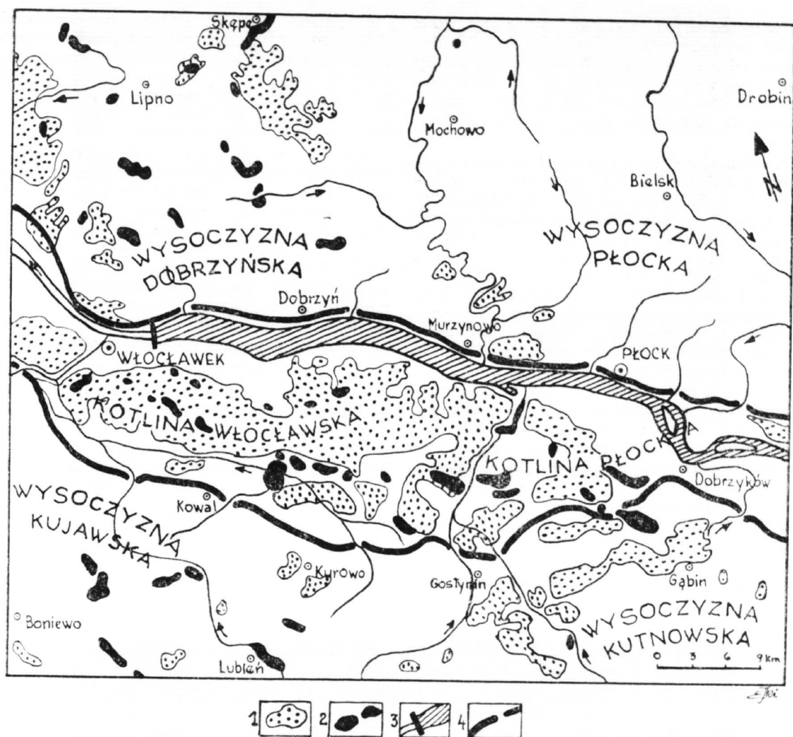
Ryc. 2 — Szkic sytuacyjny obszaru przedstawionego na obrazach satelitarnych: 1) lasy, 2) jeziora, 3) zbiornik wodny, 4) krawędź wysoczyzny.
