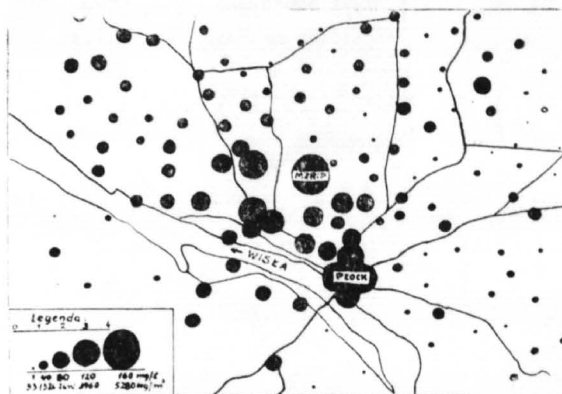
Rys. 6. Mineralizacja pokrywy śniegowej w rejonie MZRIp — PZM. Luty 1981 r. (wg W. Lenarta i W. Nowickiego, Pokrywa śnieżna jako medium do badań zanieczyszczeń dostawy zanieczyszczeń z atmosfery do gleby. Murzynowo k. Płocka).
