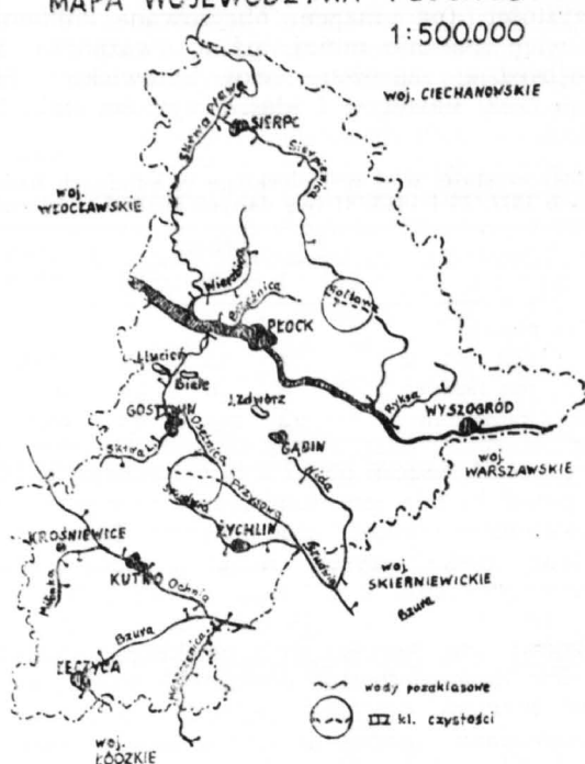
Rys. 2. Stan czystości wód województwa płockiego — rok hydrologiczny 1980/81. (wg danych OBiKS w Płocku).
