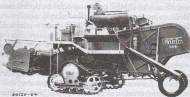
Kombajny KZB-3B w końcowej fazie produkcji w wersji do zbioru ryżu
